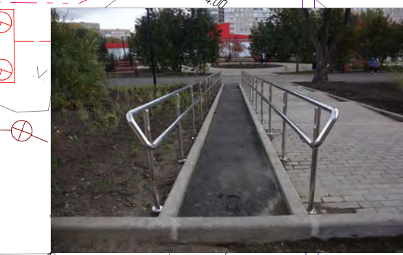
Ограждение пандуса для ММГН
